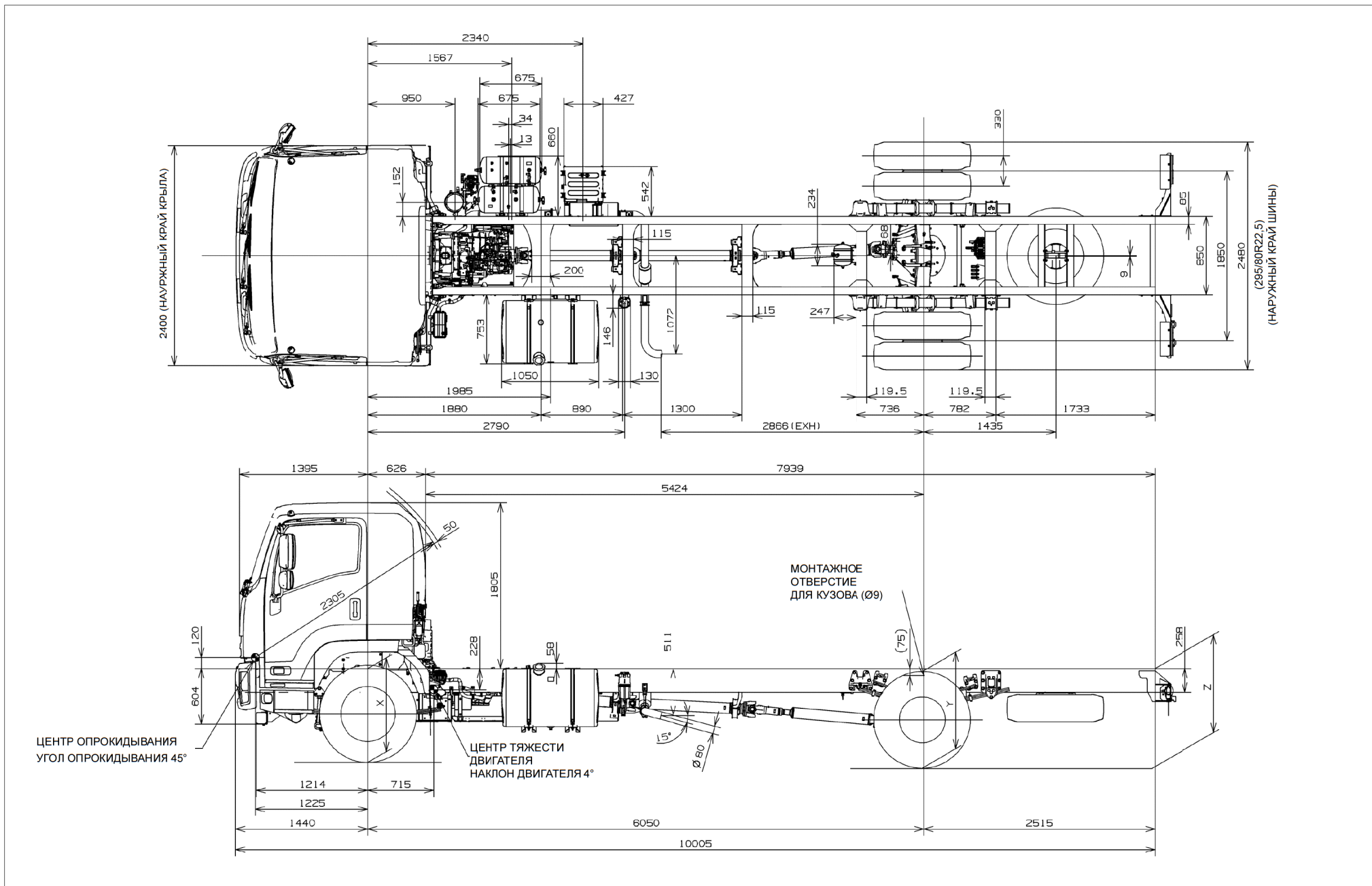
Рис. 9-1-6. Чертеж шасси с кабиной, FVR34UL-SDUC
