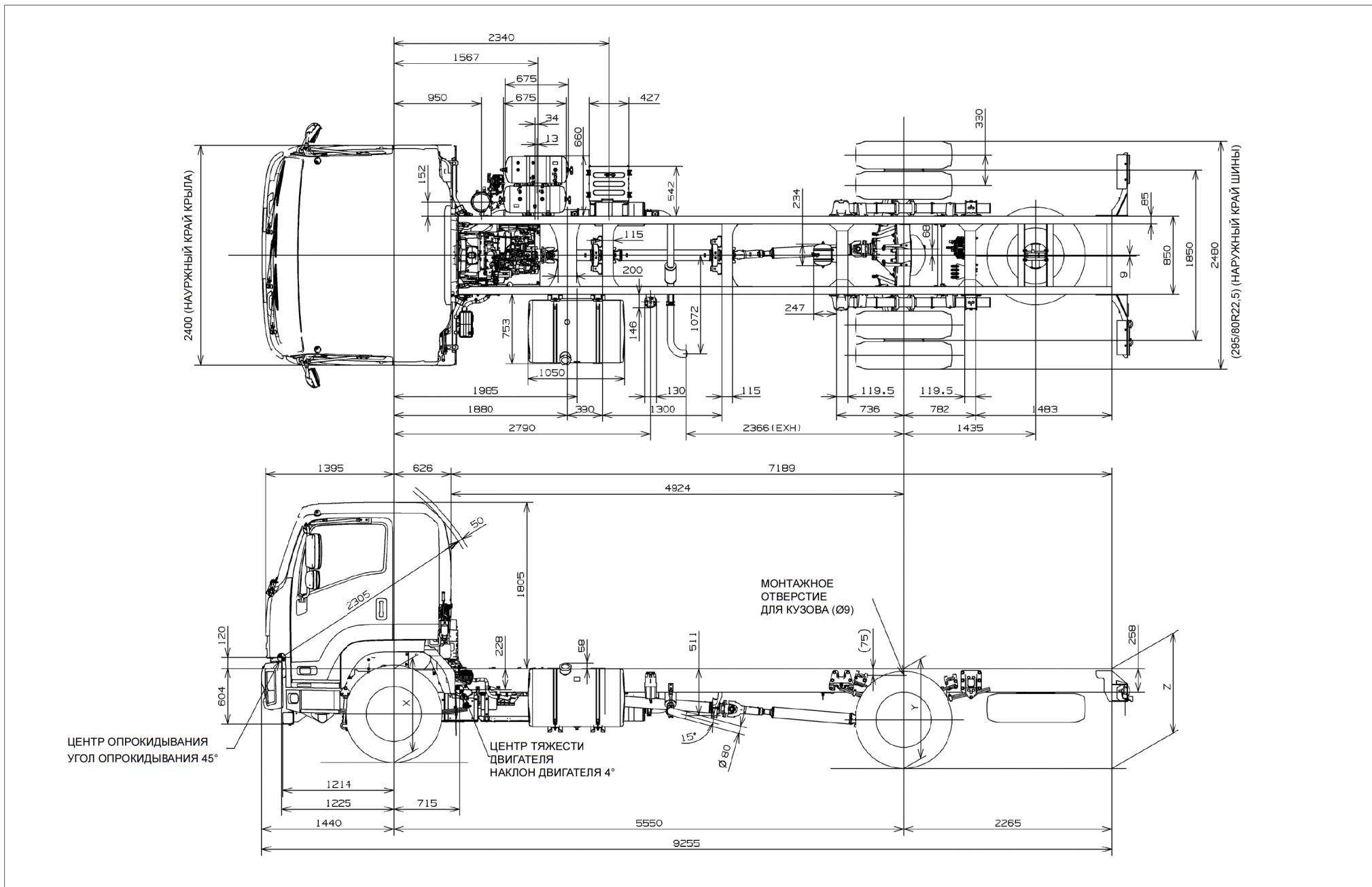
Рис. 9-1-5. Чертеж шасси с кабиной, FVR34UL-QDUC
