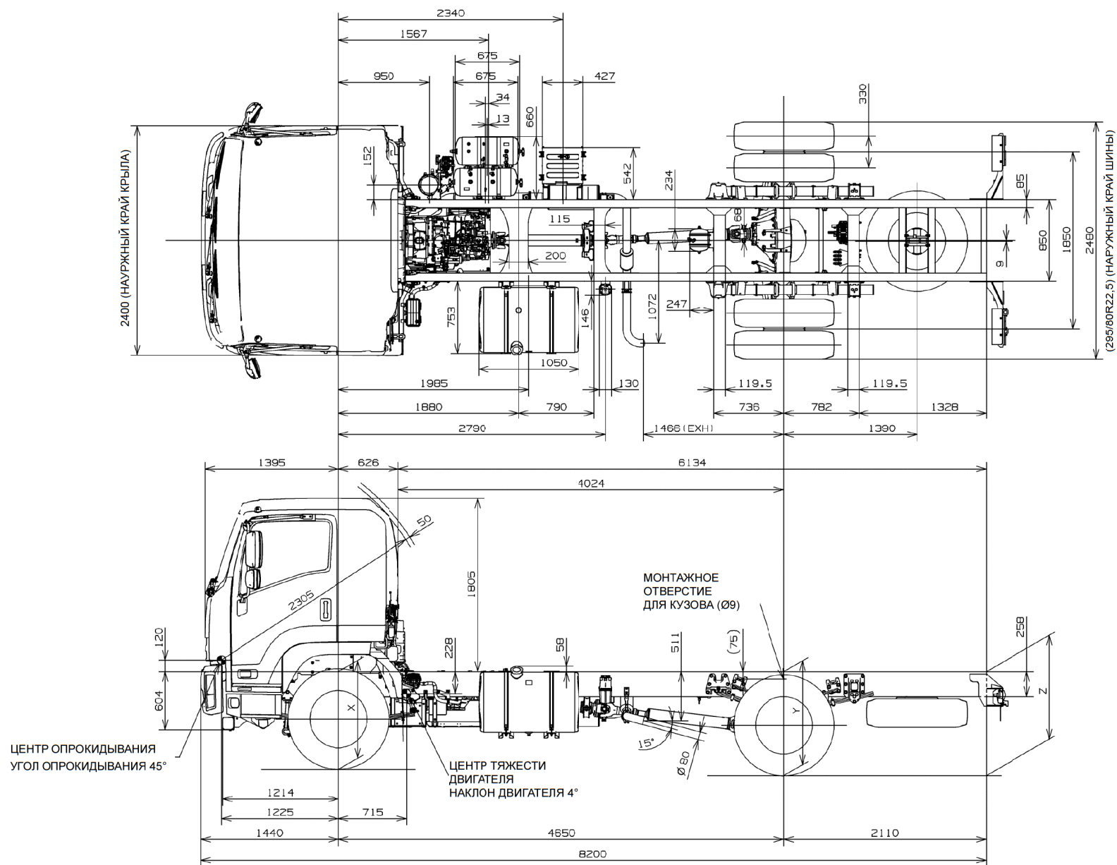
Рис. 9-1-4. Чертеж шасси с кабиной, FVR34UL-MDUC
