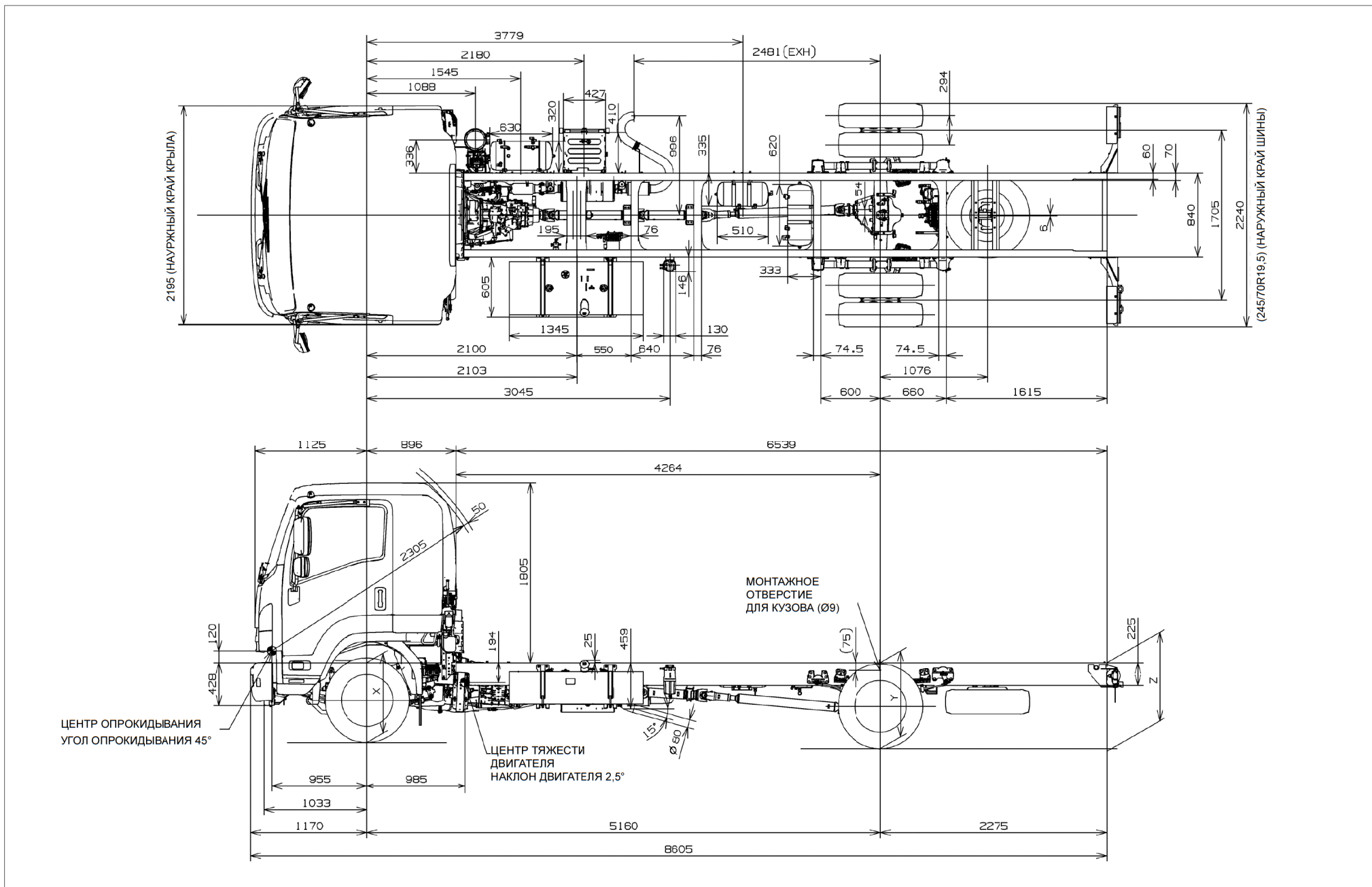
Рис. 9-1-3. Чертеж шасси с кабиной, FSR34UL-PCUN
