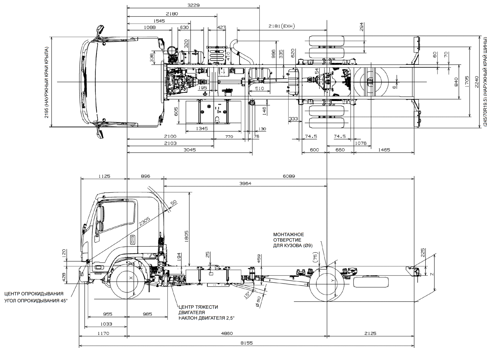
Рис. 9-1-2. Чертеж шасси с кабиной, FSR34UL-NCUN
