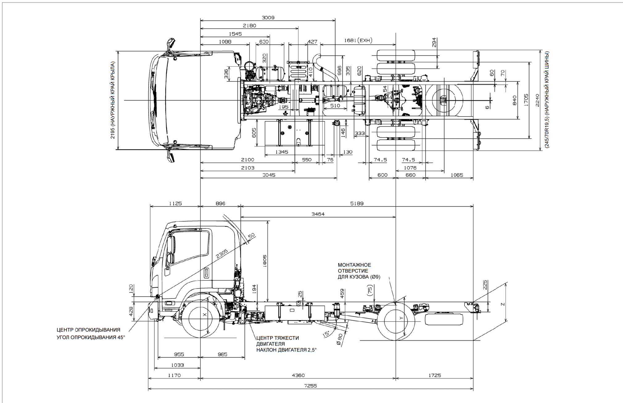
Рис. 9-1-1. Чертеж шасси с кабиной, FSR34UL-LCUN
