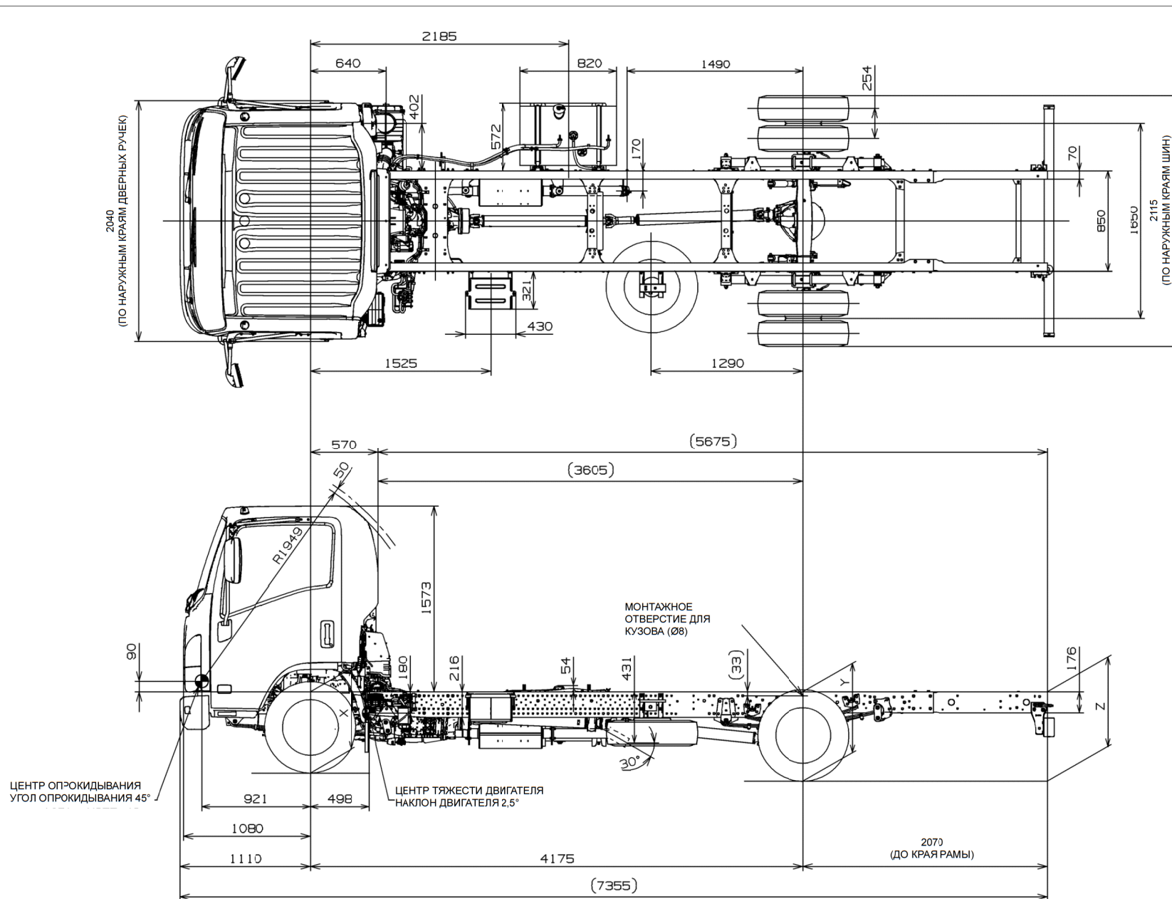
Рис. 9-1-6. Чертеж шасси с кабиной. NPR75L-LL5VAYUN
