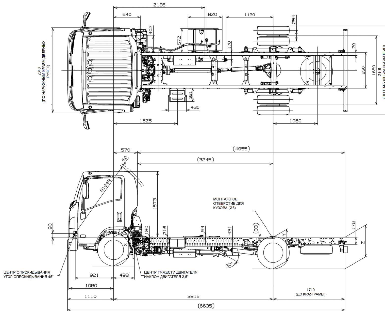
Рис. 9-1-5. Чертеж шасси с кабиной. NPR75L-KL5VAYUN
