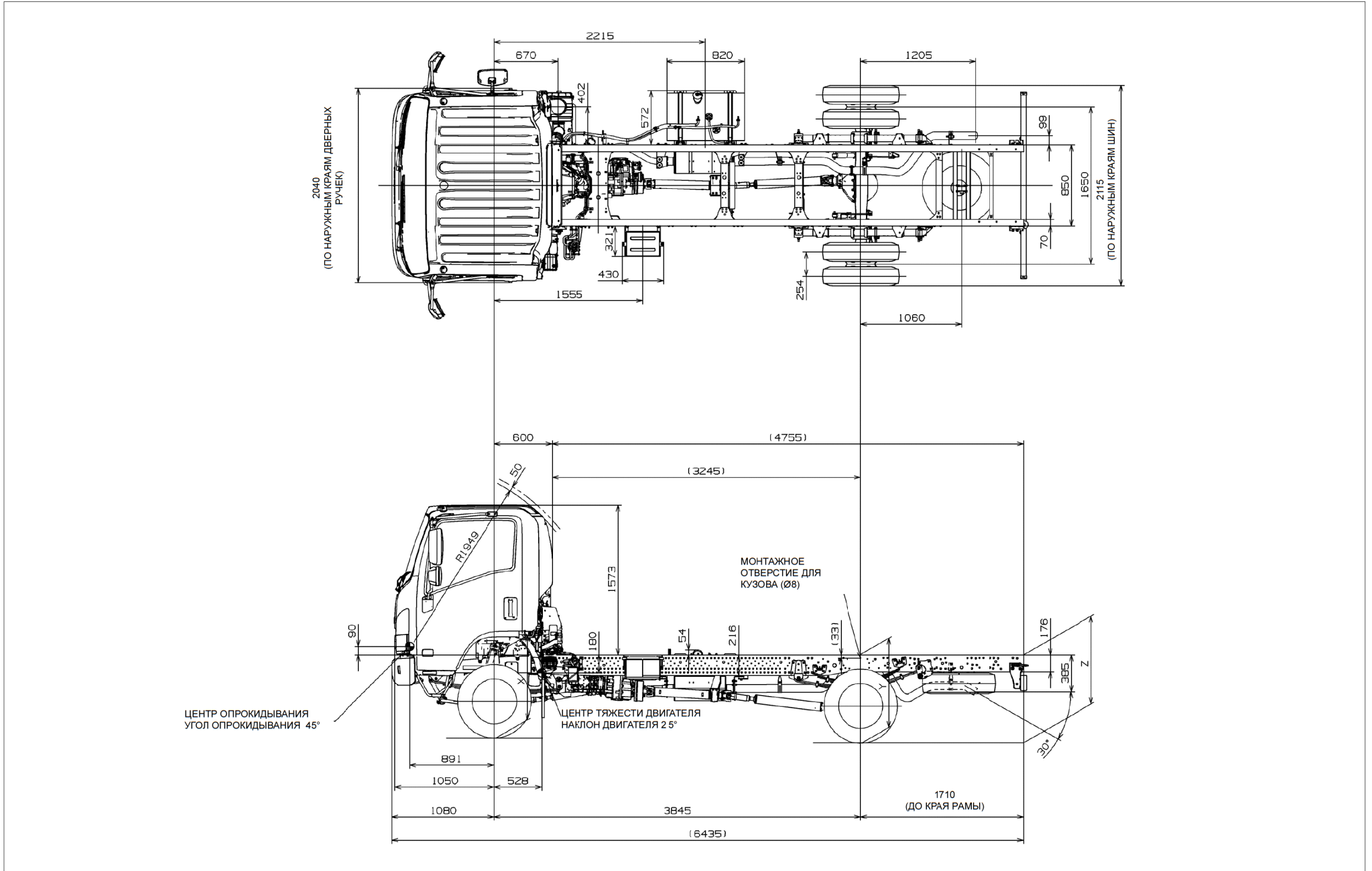
Рис. 9-1-9. Чертеж шасси с кабиной. NPS75L-KL5VAYUN
