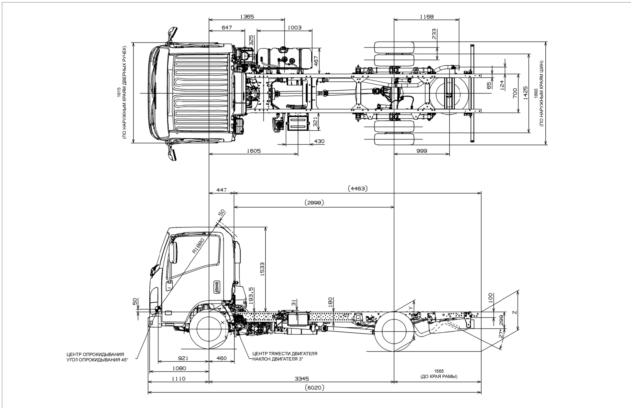
Рис. 9-1-3. Чертеж шасси с кабиной. NMR85L-НН5АУU
